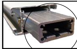
ASSEMBLAGE TENONS ÉPAISSEUR 9 mm SECTION 66 X 30 mm
